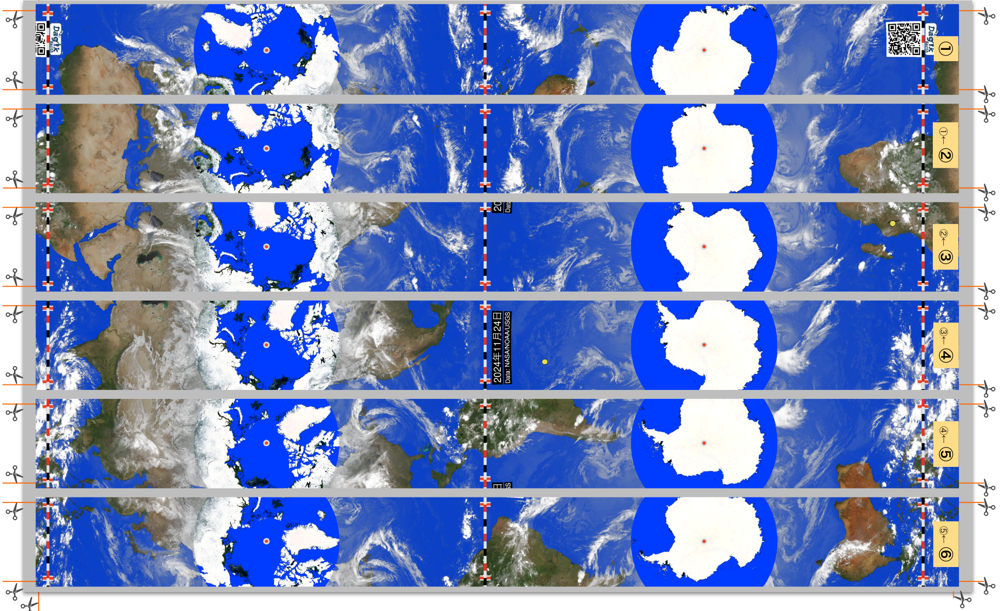
雲と地震の分布 日本が昼の12時の時に気象衛星から観測された世界中の雲の分布と、この日に発生した地震の震源の位置を示しています。 作成：ダジック・アース・プロジェクト 雲データ：「ひまわり」衛星などの静止軌道にある気象衛星による雲の観測。北極周辺と南極周辺（緯度60度以上）の地域は静止軌道からの観測が難しいため表示されていません。 TRMMプロジェクトによるNCEP/CPC 4km Global IRデータを使用しています。 雲データ提供：宇宙航空研究開発機構（JAXA） [ http://www.jaxa.jp ] 震源データ：黄色い丸マークはこの日のマグニチュード5.0以上の地震の発生場所です。 震源データ提供：U.S. Geological Survey (USGS) [ http://www.usgs.gov ] 地表画像：NASA Blue Marble: Next Generation (MODISによって撮影された地表画像)。色合いは変更しています。 地表画像提供：NASA Earth Observatory
