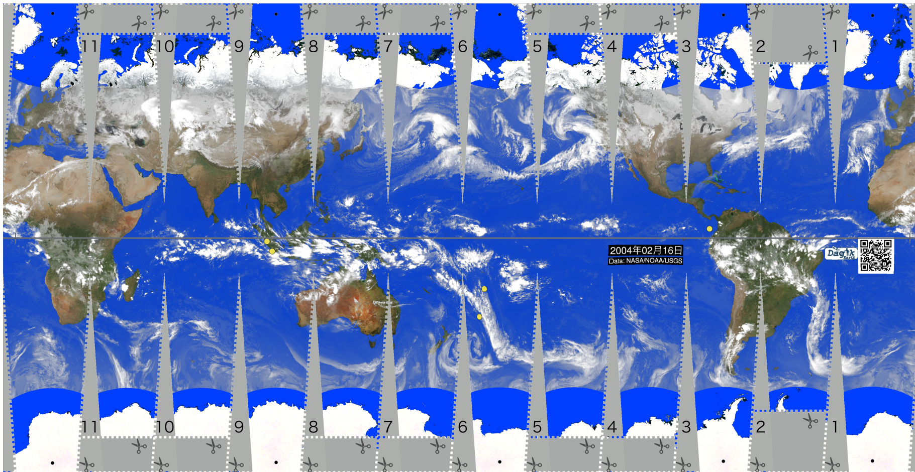
雲と地震 (M5以上) の分布
