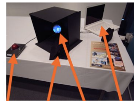
トラックボール 小型LEDプロジェクター パソコン 直径8cm発泡スチロール球
